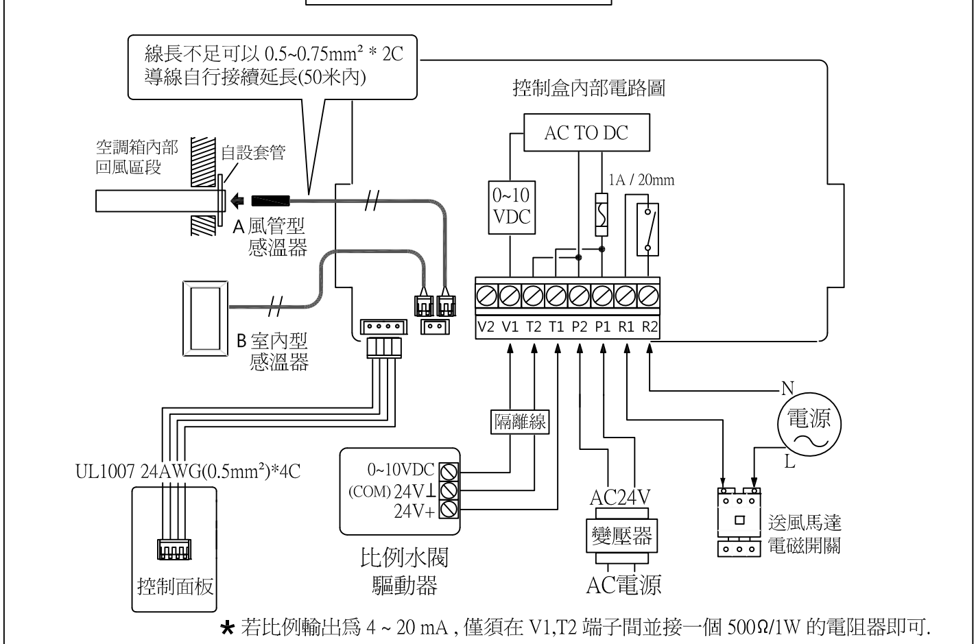
AP 比例式控制盒接線示意圖
